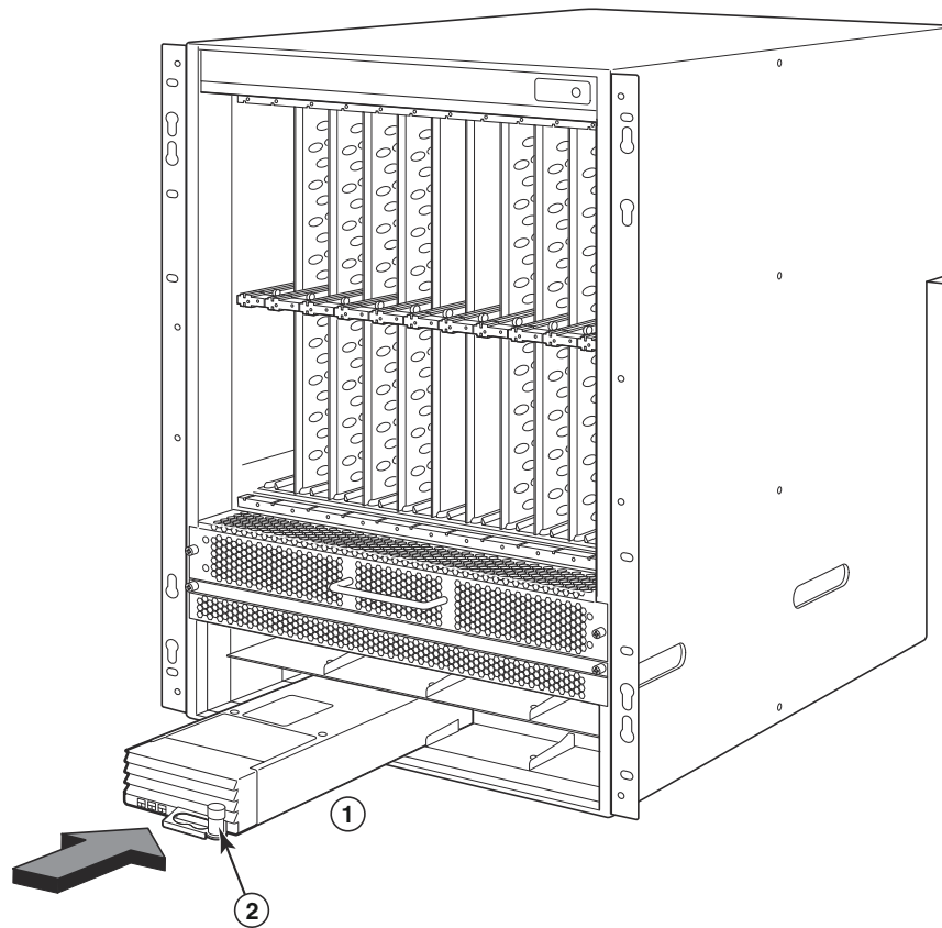
GAMBAR 87 Memasang catu daya di dalam sasis 16 slot
